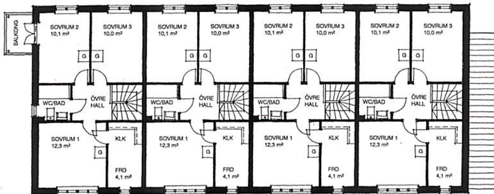
ÖVRE PLAN
